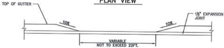
ELEVATION A-A
