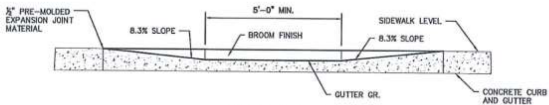
SECTION A-A
